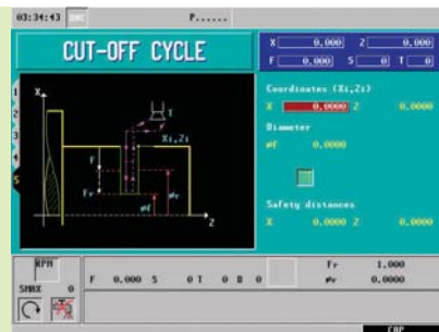
Grooving
