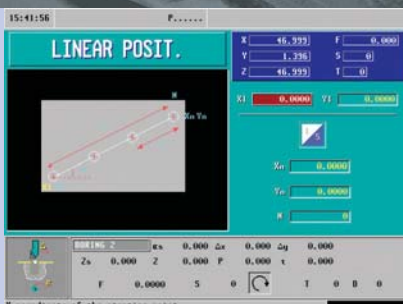
Linear positioning
